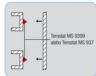
Lepenie bočných panelov, strešných alebo podlahových prvkov na nosné konštrukcie
