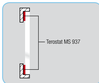
Lepenie pivičníčnych okien do kovových rámov
